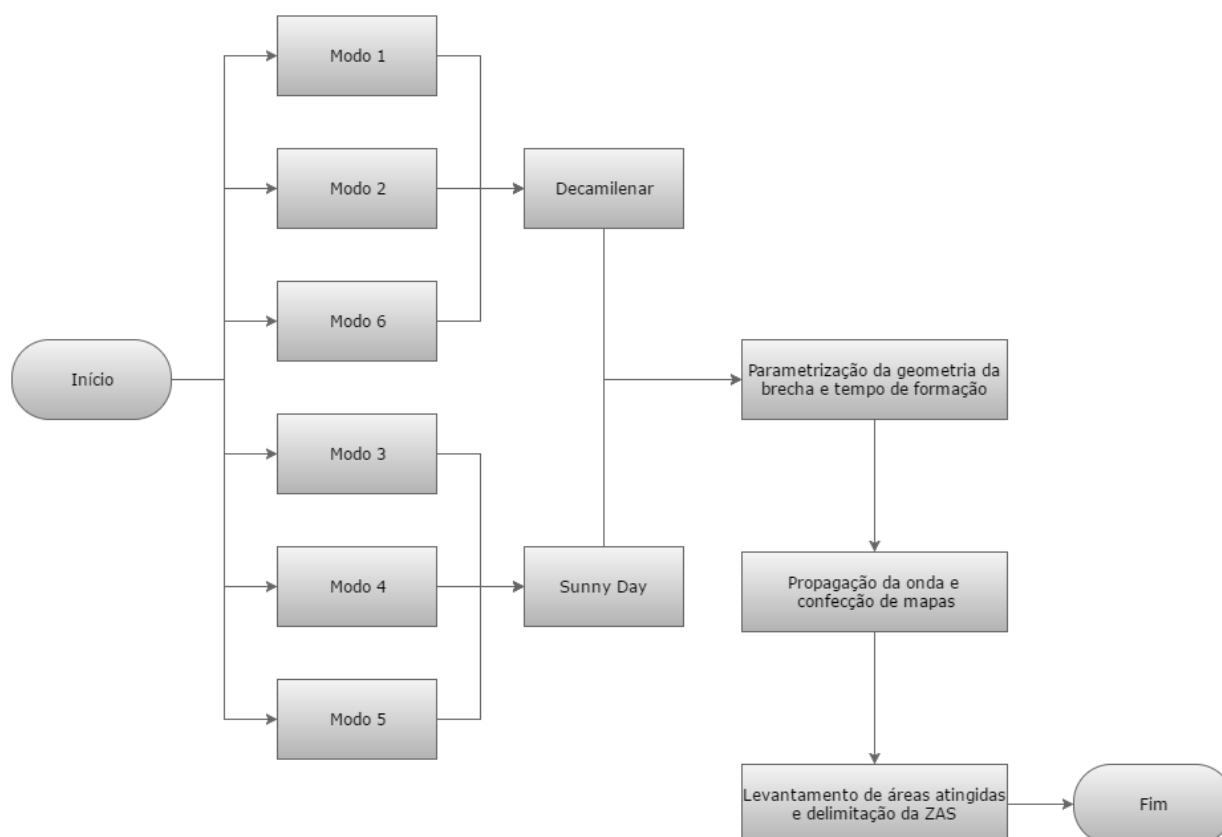
Figura 4. Cenários de ruptura da barragem Barra dos Coqueiros.
